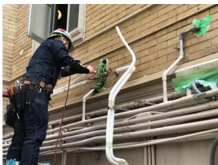
冷媒配管
